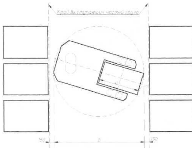
а - длина поддона с грузом; b - габариты ШТ с грузом на захвате Рисунок 4 — Параметры зазора между ПГГ и грузами
