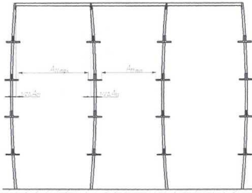
Рисунок 10 - Отклонение стоек от вертикальной плоскости внутри канала
