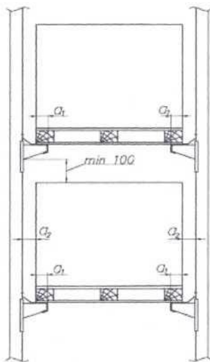
Рисунок 8 — Размещение груза относительно опорных профилей (грузонесущих направляющих)
