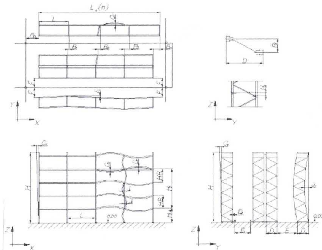
Рисунок 7 — Параметры, подлежащие контролю в не нагруженном состоянии системы
