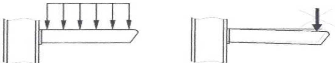
Рисунок 12 — Равно мерное распределение нагрузки по длине консоли
